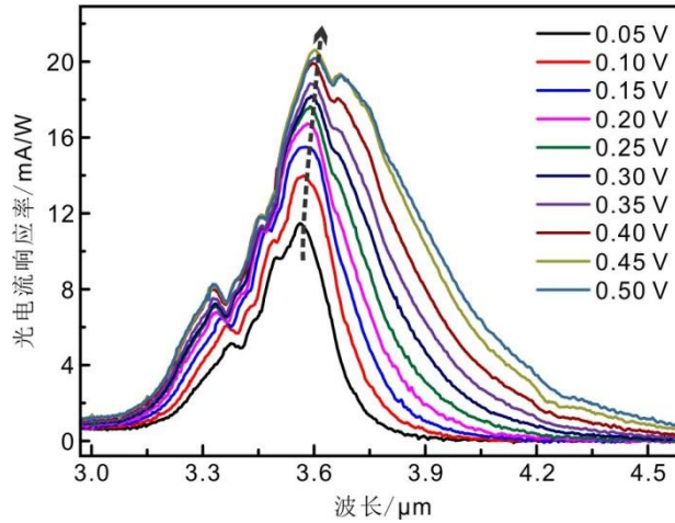
图 4 不同偏压下管状器件的光电流响应率随波长的变化关系
