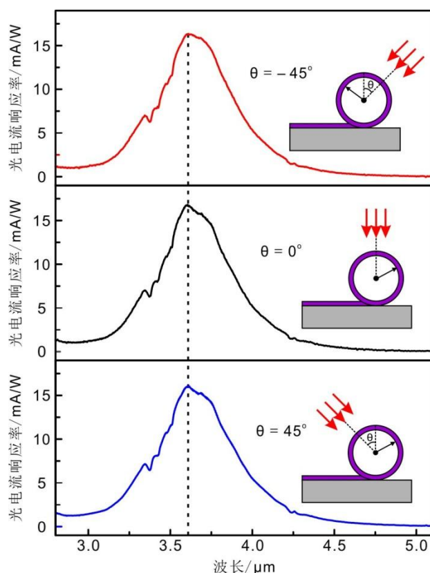
图 6 -45^\circ 、 0^\circ 和 45^\circ 入射角下管状器件的光电流响应率谱。插图为外界光的不同入射角示意图
