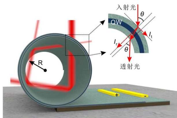
图 5 管状器件光吸收示意图。插图显示出管壁/空气界面处的光路径
