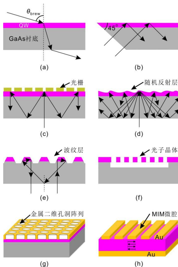
图 1 (a) 布儒斯特角耦合；(b) 45° 边耦合；(c) 光栅耦合；(d) 随机反射耦合；(e) 波纹耦合；(f) 光子晶体耦合；(g) 金属二维孔洞阵列耦合；(h) 金属-绝缘体-金属微腔耦合
